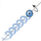
Spin do núcleo
